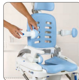
SOPORTES LATERALES ABATIBLES
